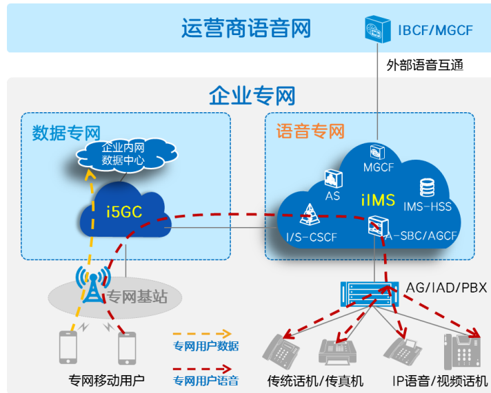
图 3-6 中兴通讯 5G 专网语音解决方案
