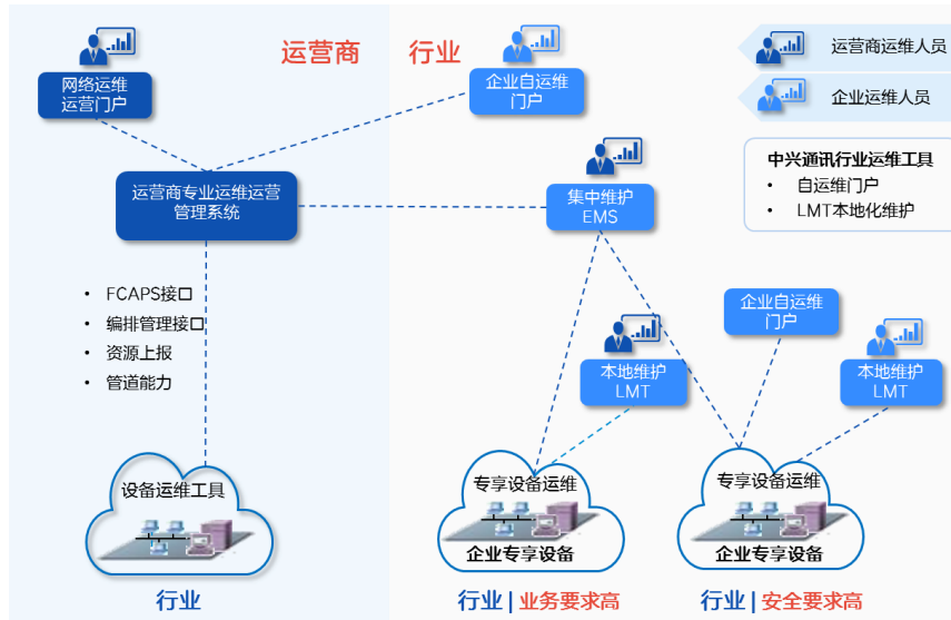
图 5-1 5G 专网“分场景”运维架构
