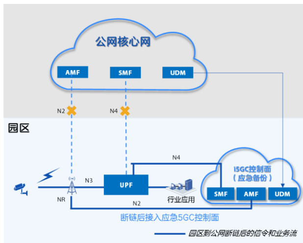
图 3-8 容灾等级 2 容灾机制
