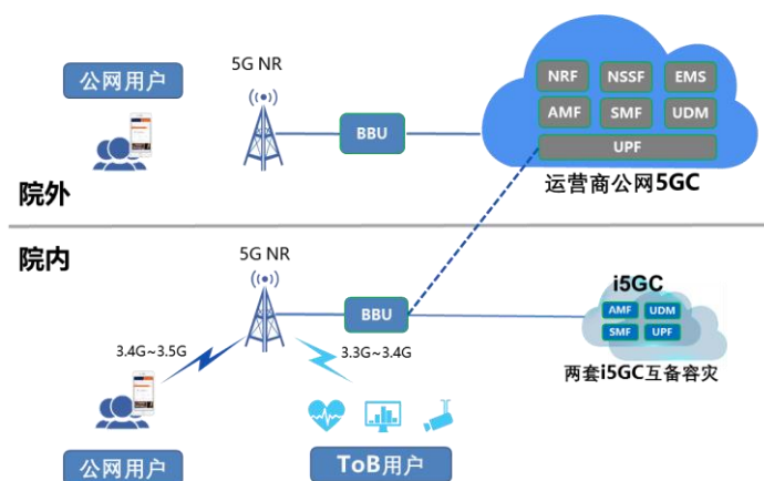
图 6-1 智慧医疗 5G 专网架构
