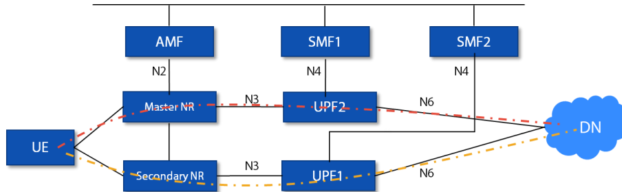
图 3-10 容灾等级 5 容灾机制
