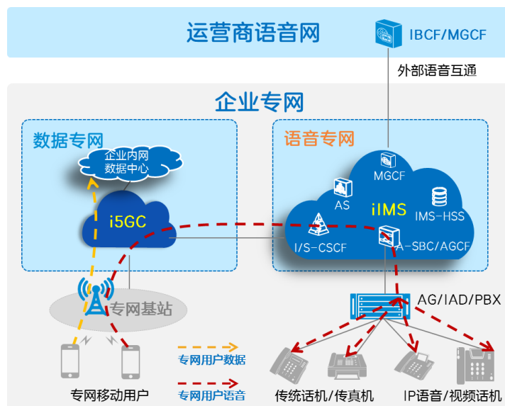
图 3-6 中兴通讯 5G 专网语音解决方案
