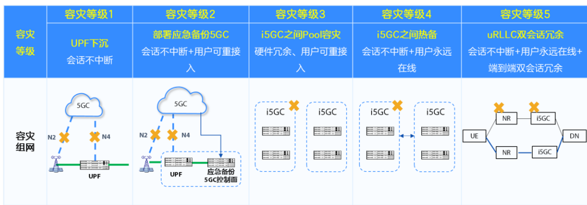
图 3-7 中兴通讯 5G 专网核心网五级容灾机制
