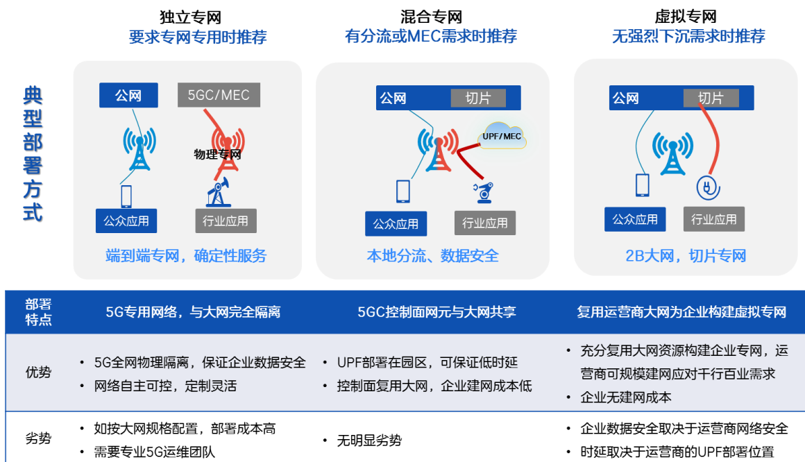
图 2-2 5G 专网部署模式及对比分析
