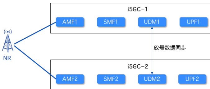
图 3-9 容灾等级 3 容灾机制
