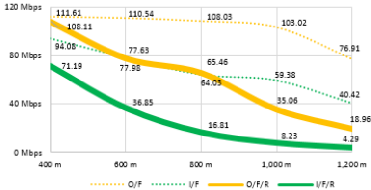
28G 综合性能 ( 叶衰&雨衰 )
