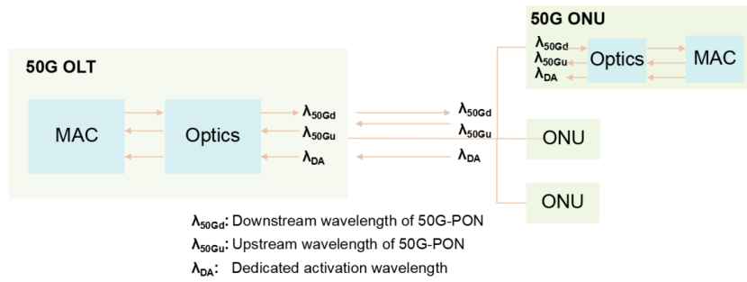
图 3-9 DAW 示例
