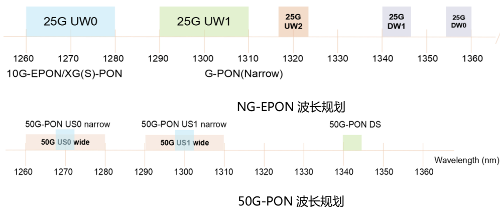
图 3-3 NG-EPON(a)和 50G-PON 波长规划选项
