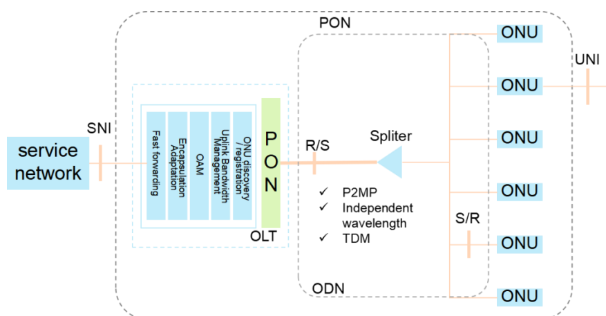
图 3-1 PON 网络架构图
