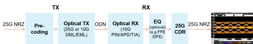
图 3-5 双二进制调制架构和信号眼图
