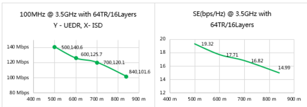
3.5G 综合性能
