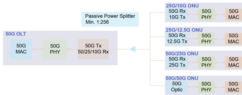
图 3-11 50G-PON 网络架构
